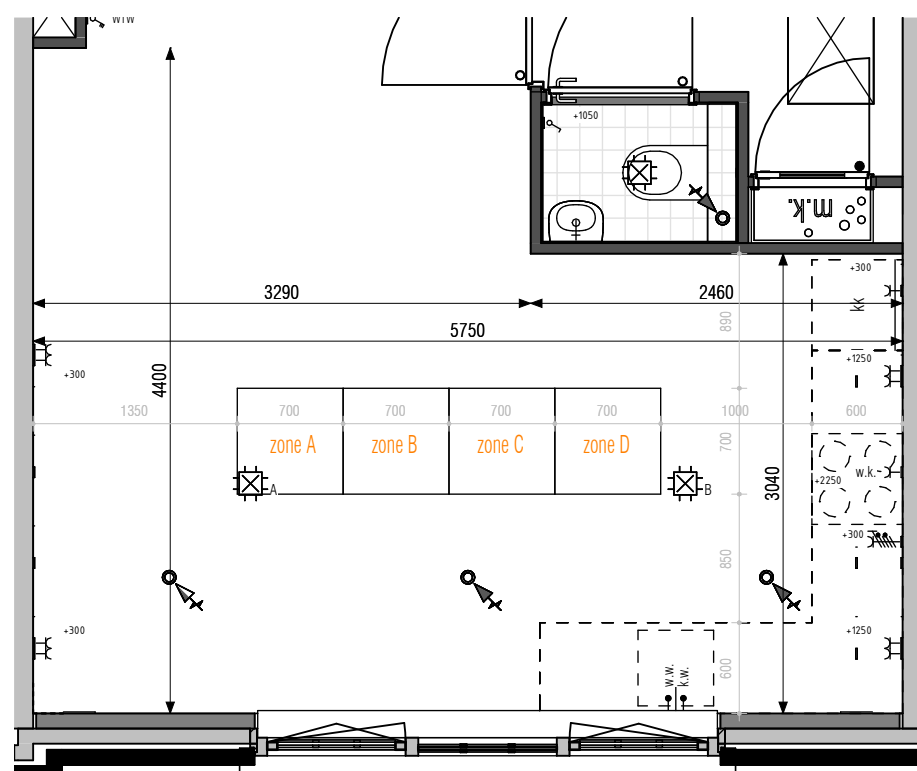
ok. vensterbank ca. 1025mm + vl.p. 476114 keukenpositie 14 LET OPI Bij keukenoptie 13, 14 en 16 kan bij een keuze van een hoge kraan, het volledig naar binnen draaien van het raam worden belemmerd. LET OPI Keukenopties 13, 14 en 16 kunnen niet gekozen worden in combinatie met een erker in de voorgevel.
