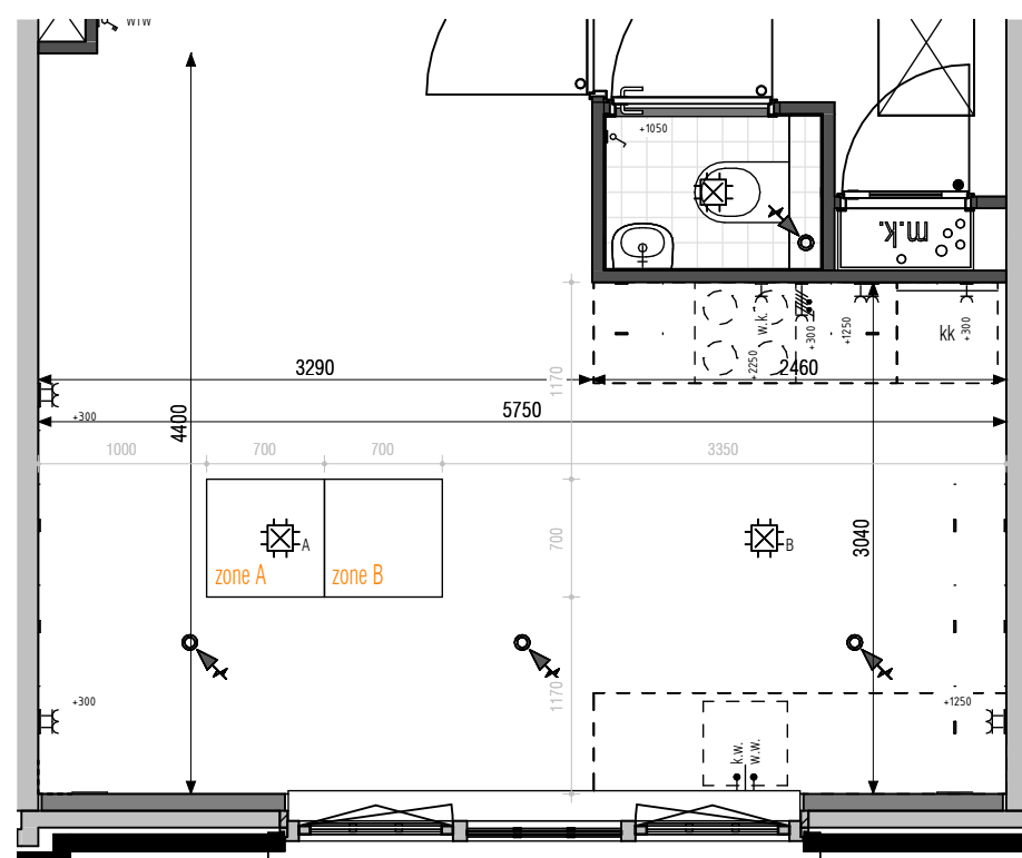
ok. vensterbank ca. 1025mm + vl.p. 476116 keukenpositie 16 LET OPI Bij keukenoptie 13, 14 en 16 kan bij een keuze van een hoge kraan, het volledig naar binnen draaien van het raam worden belemmerd. LET OPI Keukenopties 13, 14 en 16 kunnen niet gekozen worden in combinatie met een erker in de voorgevel.
