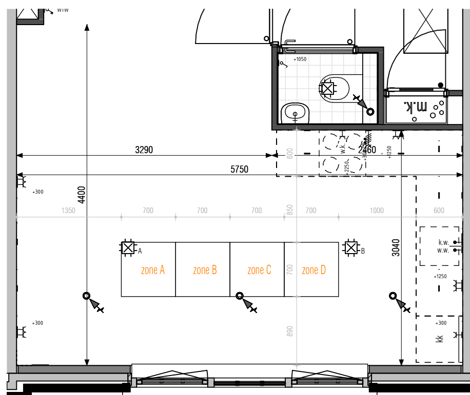
ok. vensterbank ca. 1025mm + vl.p. 476115 keukenpositie 15
