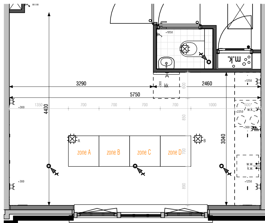
ok. vensterbank ca. 1025mm + vl.p. 476112 keukenpositie 12
