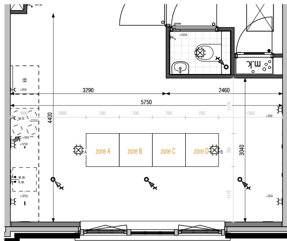
ok. vensterbank ca. 1025mm + vl.p. 476111 keukenpositie 11 (standaard)
