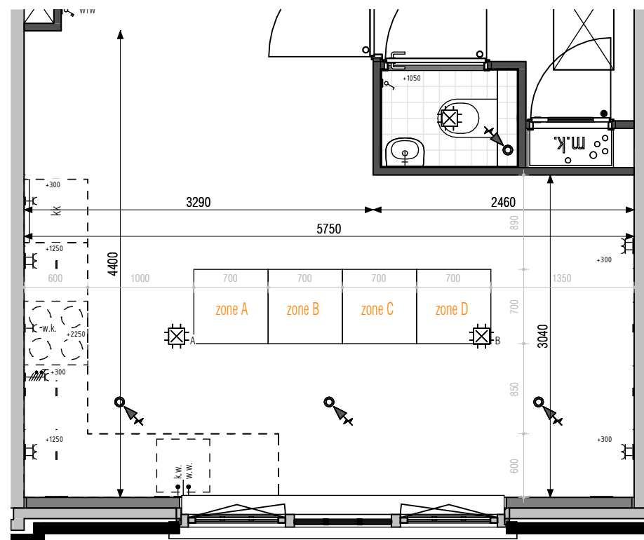
ok. vensterbank ca. 1025mm + vl.p. 476113 keukenpositie 13 LET OPI Bij keukenoptie 13, 14 en 16 kan bij een keuze van een hoge kraan, het volledig naar binnen draaien van het raam worden belemmerd. LET OPI Keukenopties 13, 14 en 16 kunnen niet gekozen worden in combinatie met een erker in de voorgevel.
