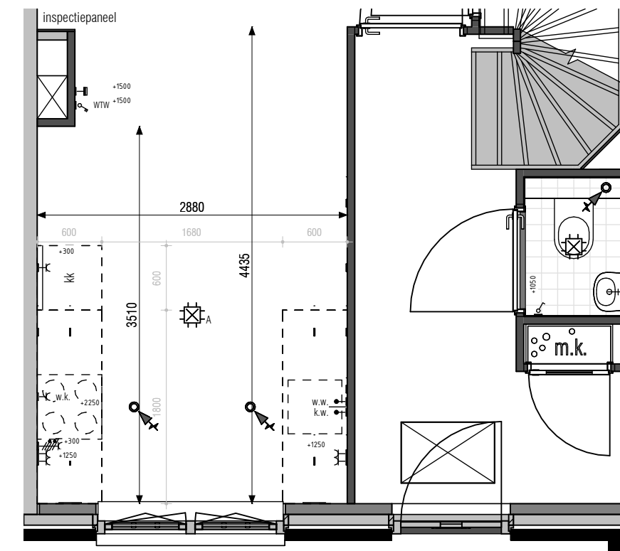
ok. vensterbank ca. 1025mm + vl.p. 475706 keukenpositie 6
