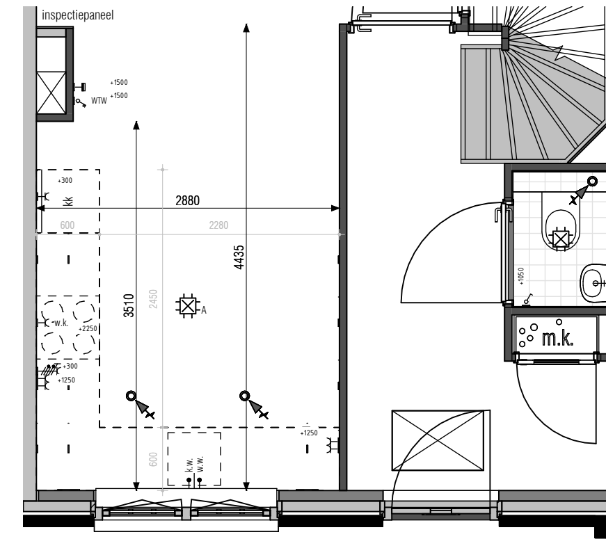
ok. vensterbank ca. 1025mm + vl.p. 475703 keukenpositie 3 LET OP! Bij keukenoptie 3 en 4 kan bij een keuze van een hoge kraan, het volledig naar binnen draaien van het raam worden belemmerd.
