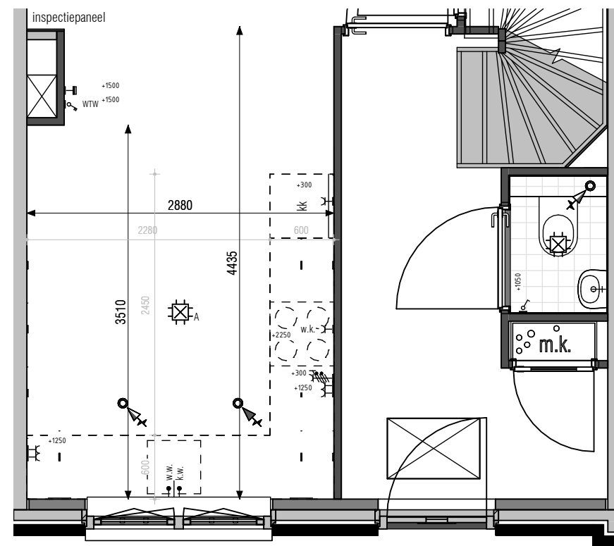
ok. vensterbank ca. 1025mm + vl.p. 475704 keukenpositie 4 LET OP! Bij keukenoptie 3 en 4 kan bij een keuze van een hoge kraan, het volledig naar binnen draaien van het raam worden belemmerd.
