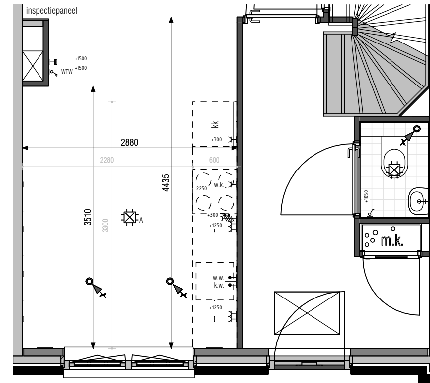
ok. vensterbank ca. 1025mm + vl.p. 475702 keukenpositie 2
