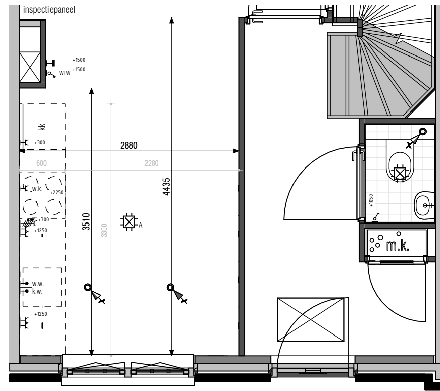
ok. vensterbank ca. 1025mm + vl.p. 475701 keukenpositie 1 (standaard)
